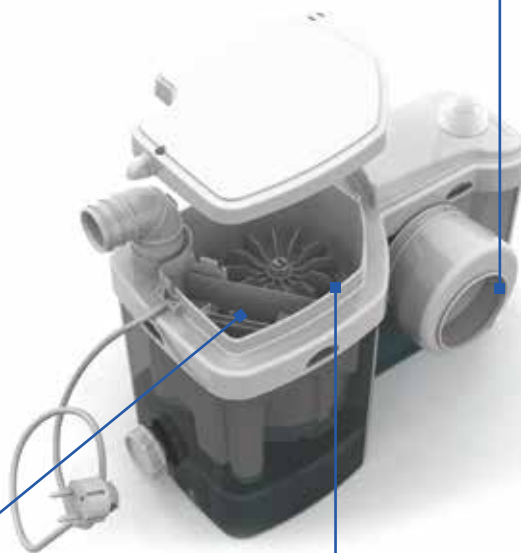
Double cuve permettant une intervention facile et rapide en milieu sec
